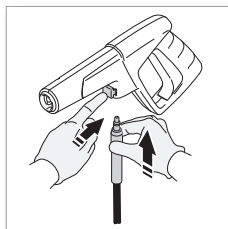
5. Poussez pour attacher le tuyau à haute pression au pistolet de pulvérisation.
